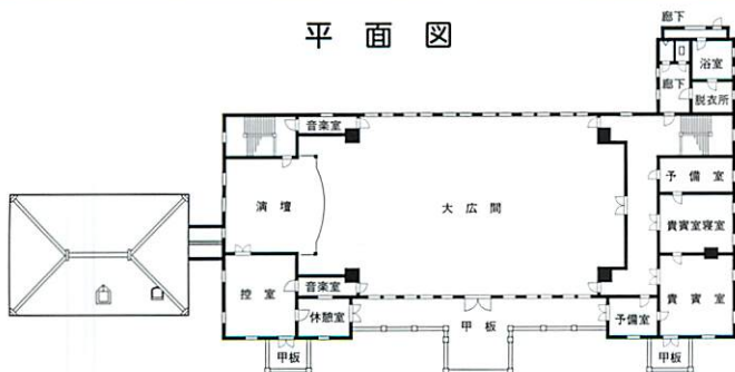
旧函館区公会堂二階平面図
