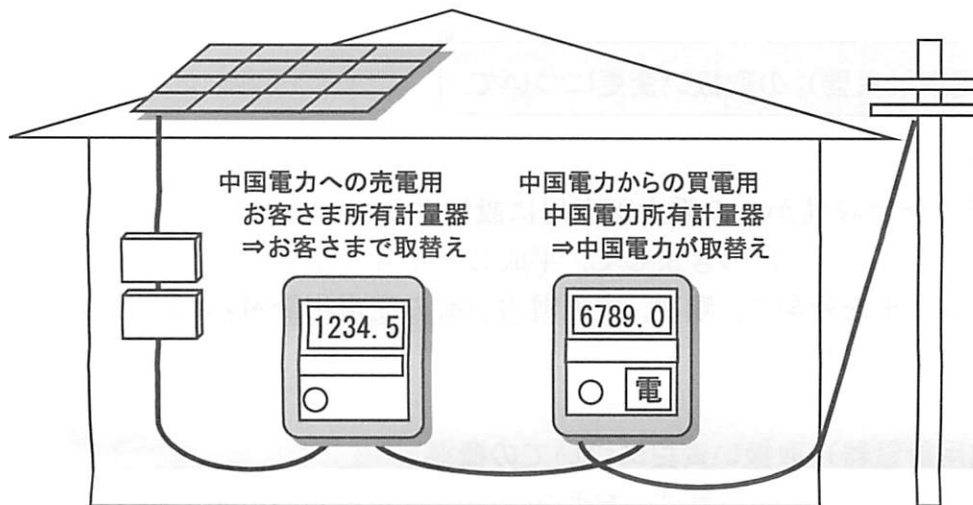
これまでの計量器設置イメージ
